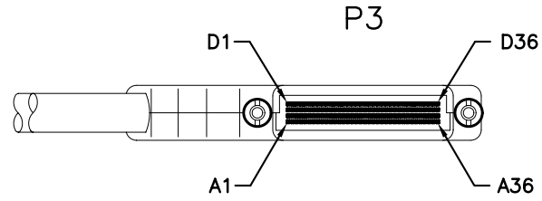
RECEPTACLE
