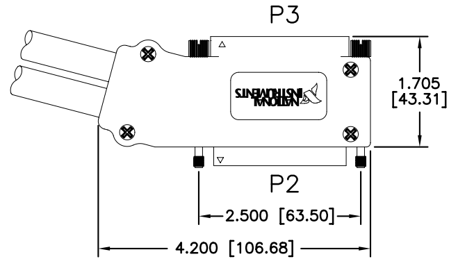
RECEPTACLE
